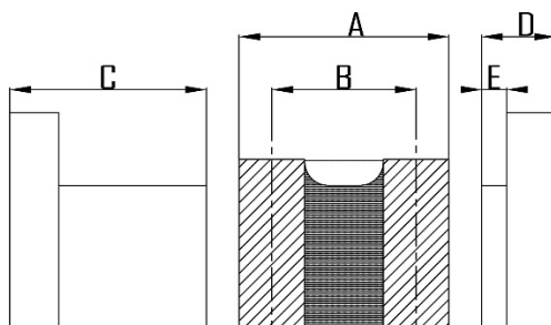
Рисунок 5 - Контрольные точки износа тормозных колодок и тормозного диска
