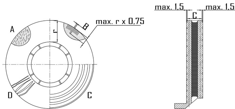
Рисунок 6 - Возможные трещины на тормозном диске
