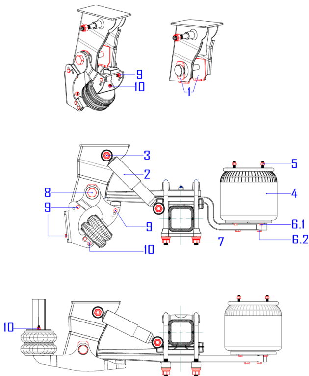
Рисунок 9 - Контрольные точки системы пневматической подвески
