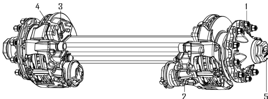
Рисунок 8 - Точки затяжки
