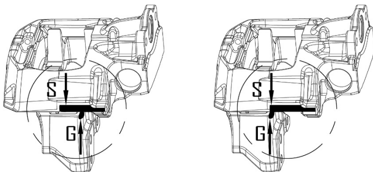
Рисунок 4 - Проверка толщины колодок дискового тормоза
