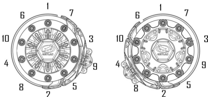
Рисунок 3 - Рекомендуемая последовательность затяжки колесных гаек
